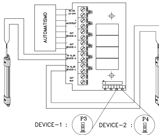
Cableado de 1 dispositivo por canal Wiring of 1 device per channel
