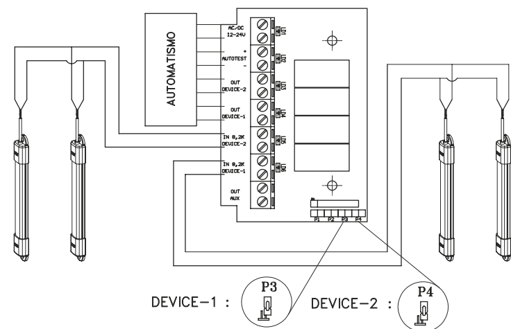
Cableado de 2 dispositivos por canal (max.) Wiring of 2 devices per channel (max allowed).
